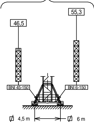
(H) TRASLACIÓN / TRAVELLING / TRASLATION / ПЕРЕМЕЩЕНИЕ / RAY YÜRÜYÜŞLÜ / متحركة
